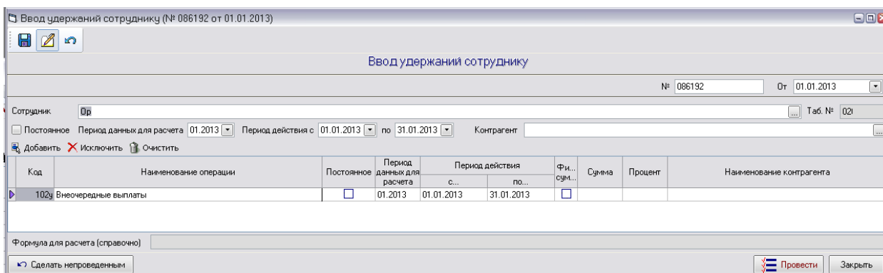
Рис. 2-92 Окно «Ввод удержаний сотруднику»
